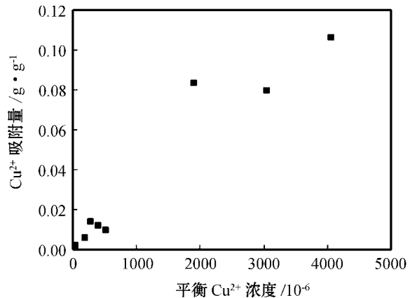
图 4 施氏矿物对 \text{Cu}^{2+} 的吸附等温线
