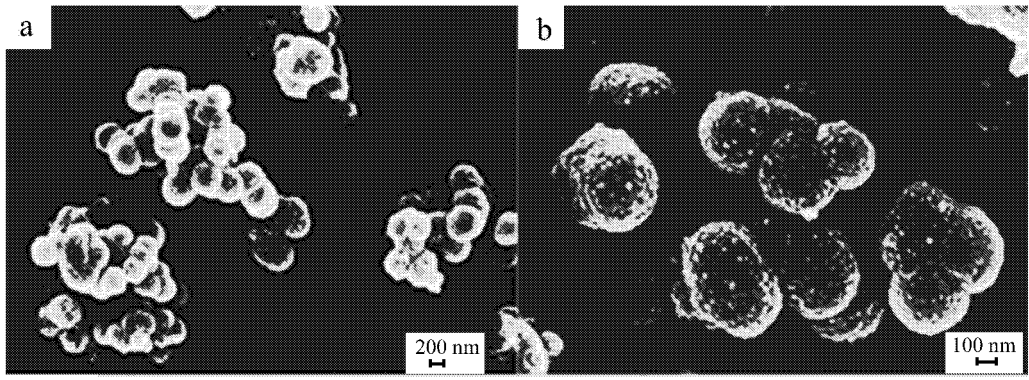
图 2 施氏矿物的 SEM 照片
