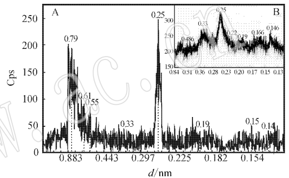
图 1 施氏矿物 XRD 衍射图谱
