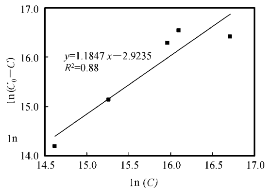
图 8 施氏矿物吸附 A. f. 的 Freundlich 模型拟合
