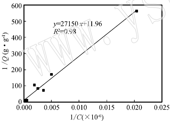
图 5 施氏矿物吸附 \text{Cu}^{2+} 的 Langmuir 模型拟合
