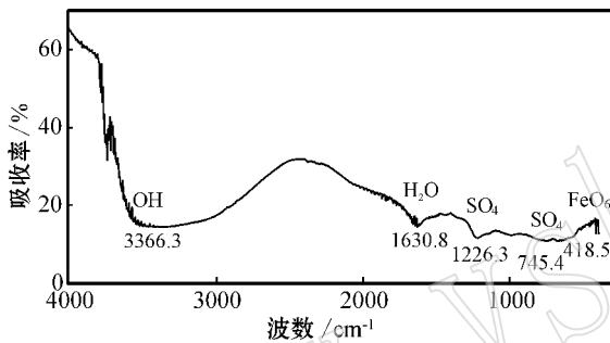
图 3 施氏矿物红外光谱图
