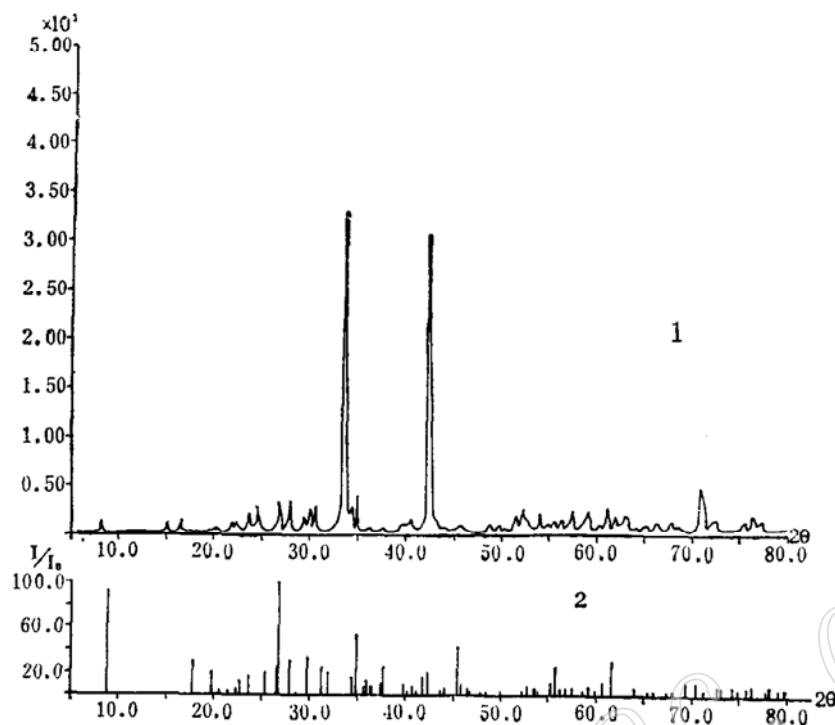
图1 南平石的X射线粉末衍射图谱(工作条见表2)
