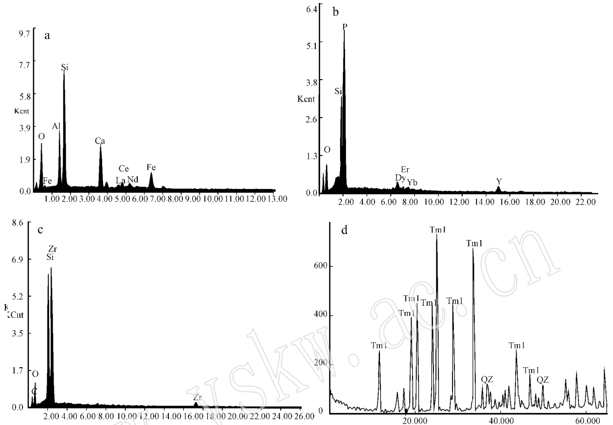
图 3 电子探针能谱图及 XRD 衍射谱图
