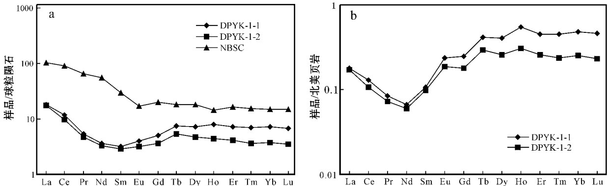
图 4 电气石岩标准化稀土元素配分模式图
