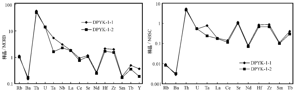
图5 电气石岩微量元素蛛网图
