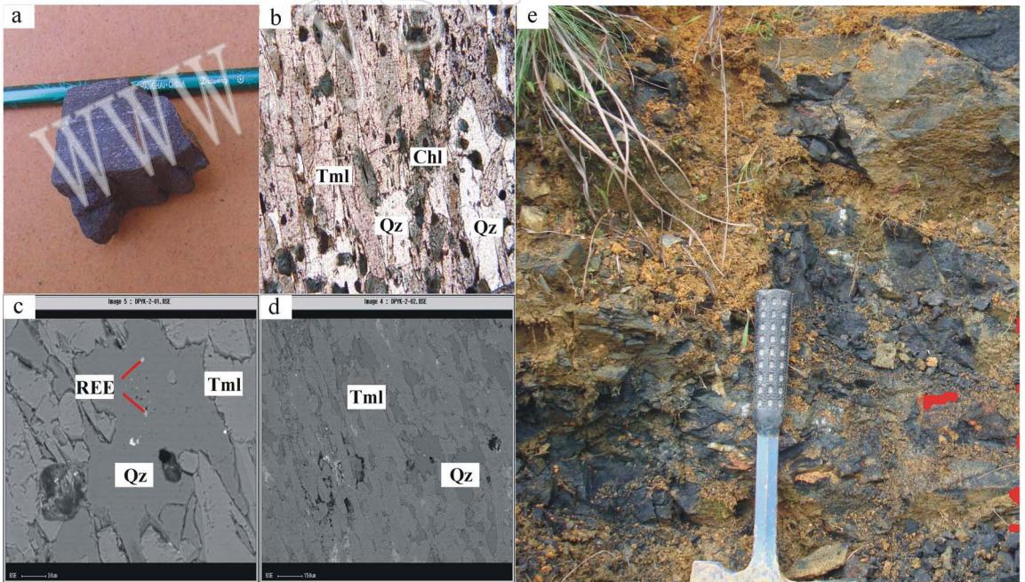
图 2 电气石岩的照片
