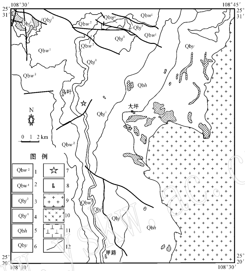
图 1 贵州大坪矿区区域地质简图(据 1:200 000 区调资料修改) ①
