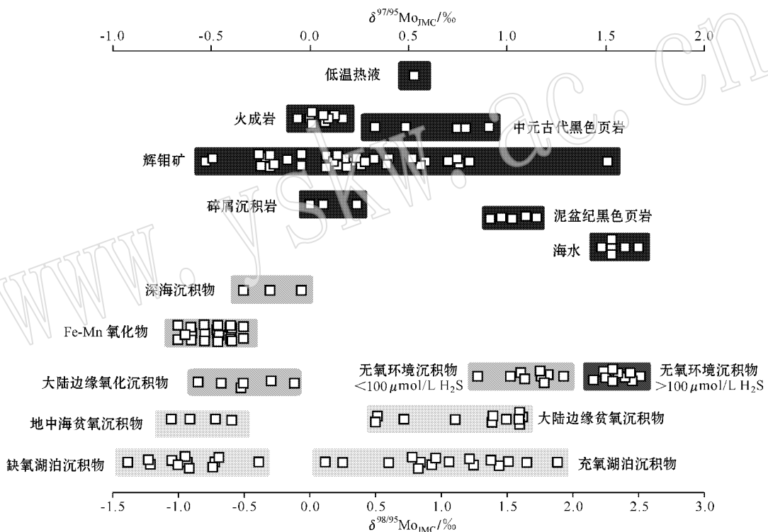
图 1 自然界中 \text{Mo} 同位素组成变化图[数据引自 Siebert 等( 2003 )、Barling 和 Anbar( 2004 )、Anbar 和 Rouxel( 2007 )、Malinovsky 等( 2007a, 2007b )]
