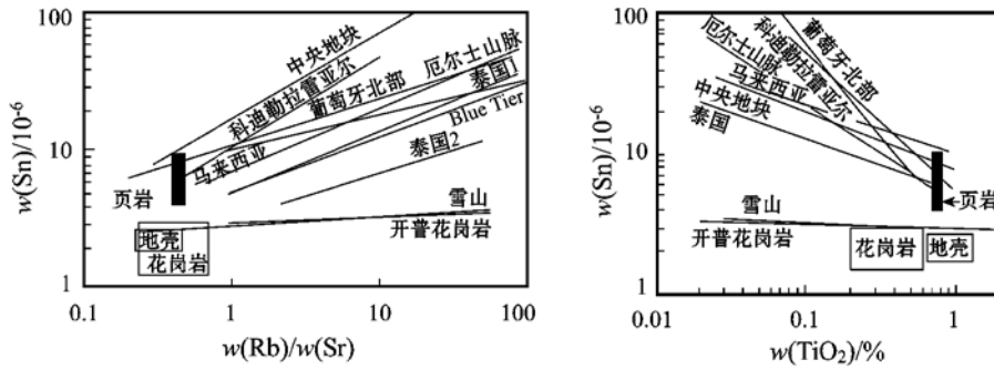
图 3 世界成 Sn 花岗岩的 Sn- TiO 2 和 Sn- Rb/Sr 图解 (据 Lehmann, 1990)
