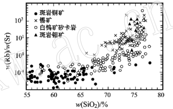
图 2 不同背景下矿化花岗岩的 Rb/Sr- SiO_2 图解 (据 Blevin 和 Chappell, 1995)
