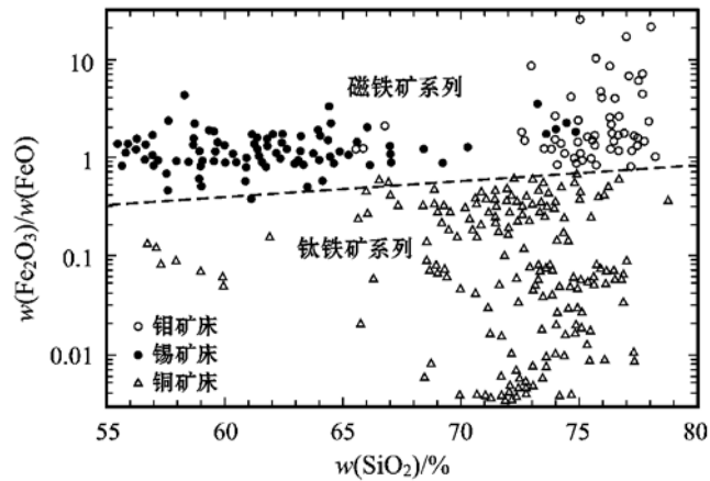
图 5 与 Cu、Mo、Sn 矿床有关的花岗岩 SiO_2 - Fe_2O_3/FeO 变异图 (据 Lehmann, 1990)
