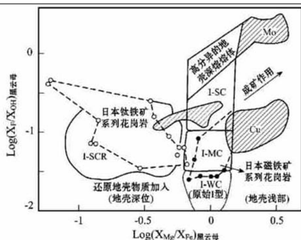
图 6 I 型花岗岩黑云母成分分类及与斑岩有关的 W、Mo、Cu 矿床中的热液黑云母的对标 (据 Brimhall 等, 1988)
