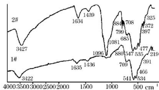
图4 样品的IR图谱
