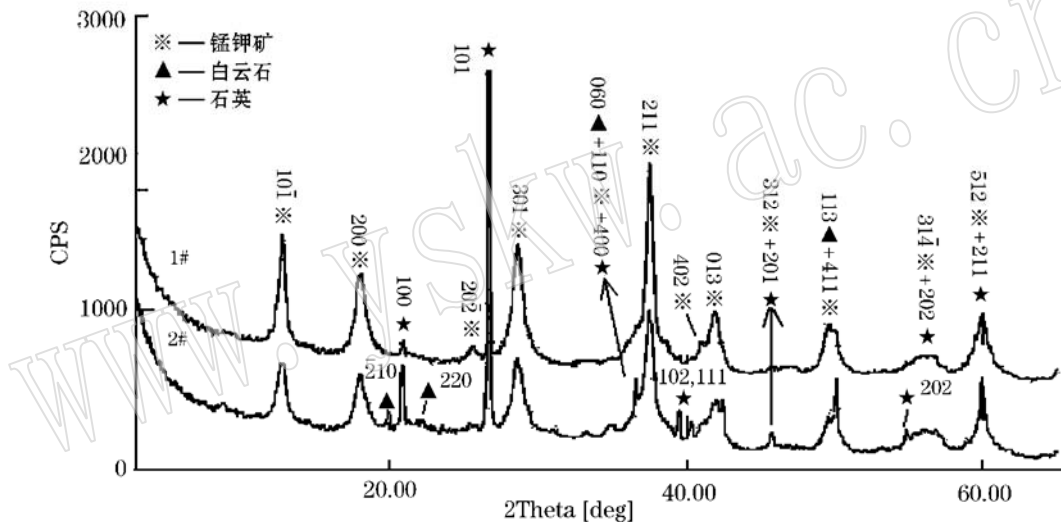
图3 样品的XRD图谱
