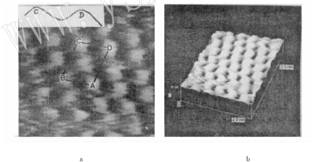
图 4a 辉锑锡铅矿 {100}解理面的 STM 图像
