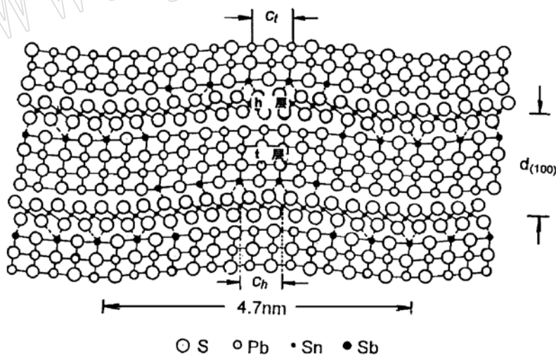
图1 辉锑锡铅矿晶体结构模型沿[010]方向的投影(汪苏,1992)
