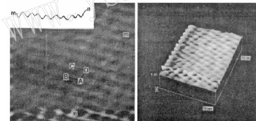
图 7a 辉锑锡铅矿 {100}解理面的 STM 图像
