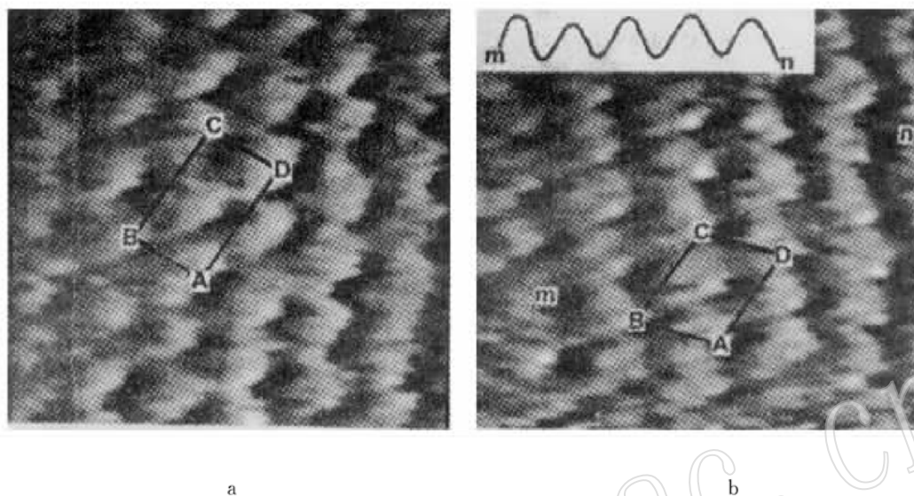
图 3 辉锑锡铅矿 {100}解理面的 STM 图像
